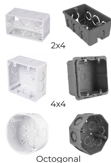
Cajas de empalme
